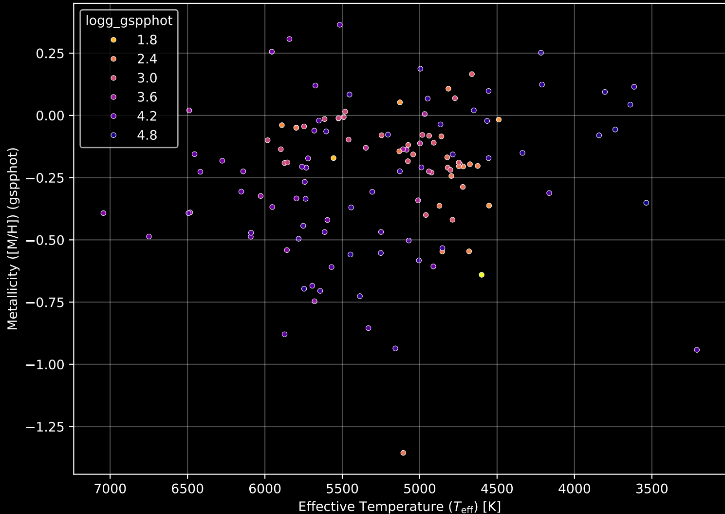
APOGEE DR17 Field: [046+48_MGA] Stellar Population Parameters (n= 129)
